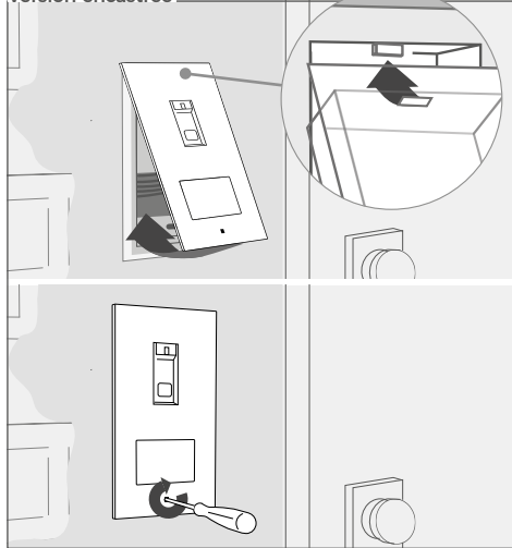
Version encastrée
