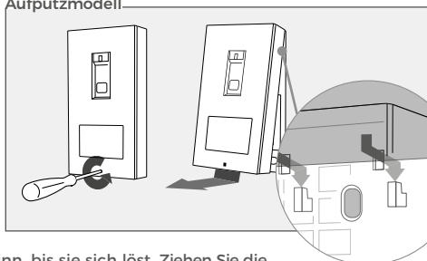
Aufputzmodell
