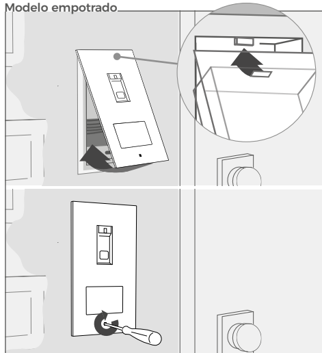
Modelo empotrado
