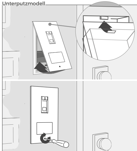
Unterputzmodell
