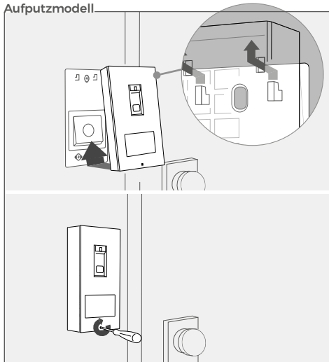
Aufputzmodell
